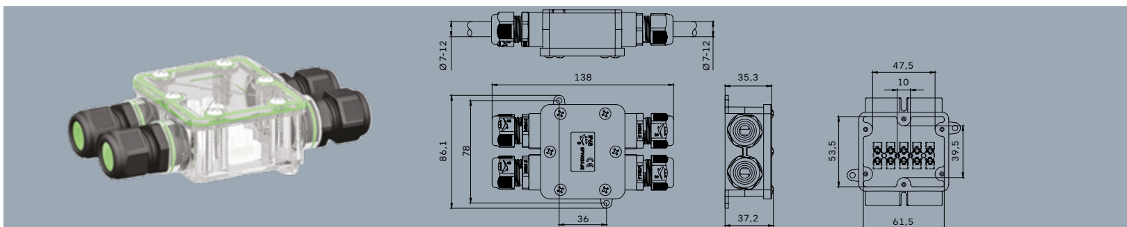
Κωδ. 020777 Κουτί σύνδεσης IP68 (EPW024.68)
