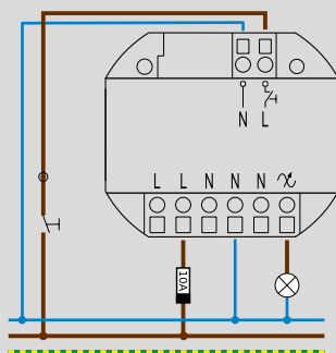
Διάγραμμα συνδεσμολογίας
