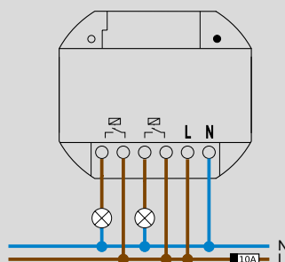
Διάγραμμα συνδεσμολογίας
