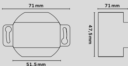
Σχέδιο / Διαστάσεις
